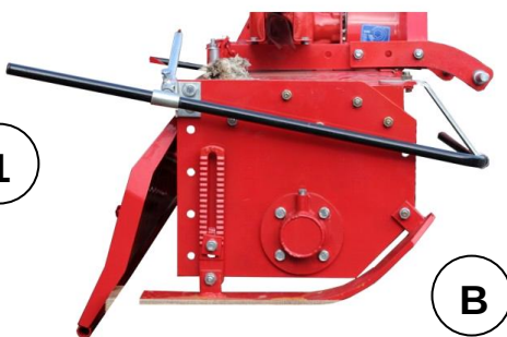
Slika 15. Podešavanje sa desnom papučom
