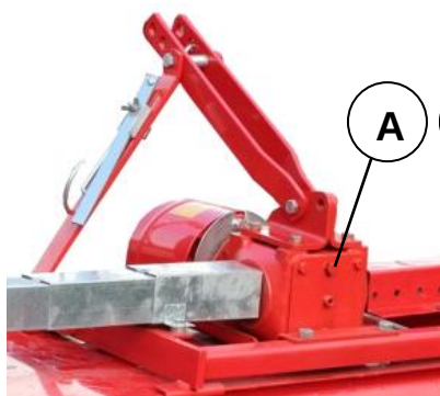
Slika 13. Kućište reduktora A - Otvor za nalivanje ulja B - Otvor za kontrolu nivoa ulja C - Otvor za ispuštanje ulja
